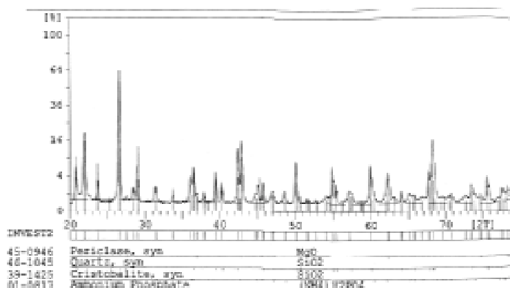
شکل ۴: الگوی پراش پرتو ایکس (XRD) و آنالیز فازي اینوستمنت
