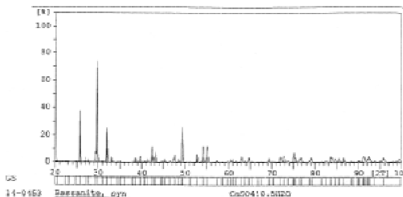
شکل ۶: الگوی پراش پرتو ایکس (XRD) آنالیز فازي استون توليدي
