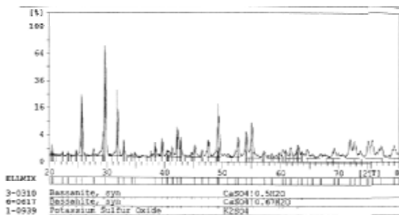
شکل ۱: الگوی پراش پرتو ایکس گچ ول میکس
