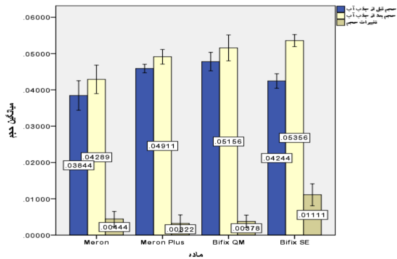
نمودار ۴: میانگین انبساط ناشی از جذب آب ۴ گروه سمان بر حسب سانتی‌متر مکعب
