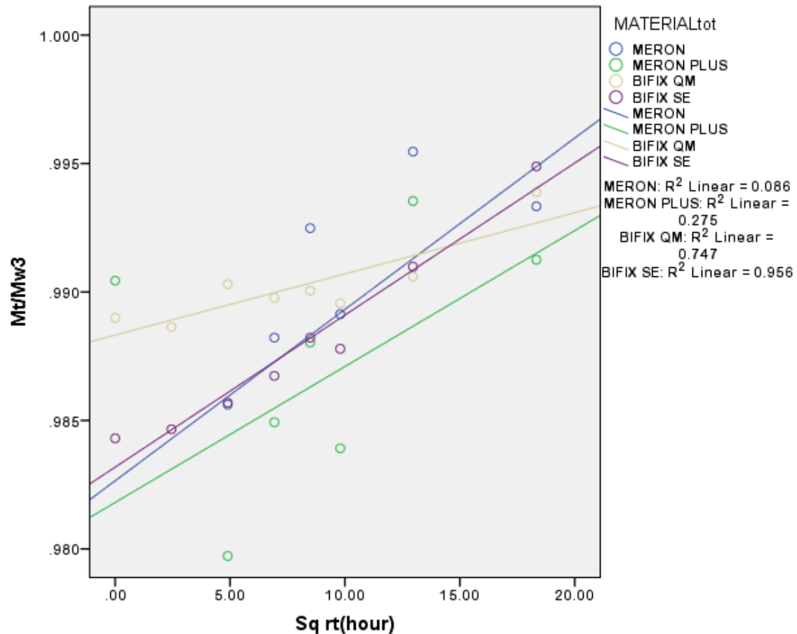
نمودار ۳. مقایسه‌ی بین منحنی‌های مربوط به نسبت جرم در زمان t به جرم در زمان بی‌نهایت در مقابل جذر زمان چهار سمان
